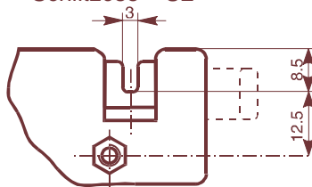
Schlitzöse " U2 "
